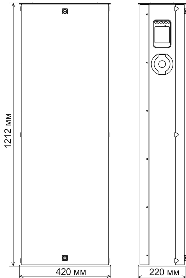
Рисунок 1 – Габаритный чертеж станции
