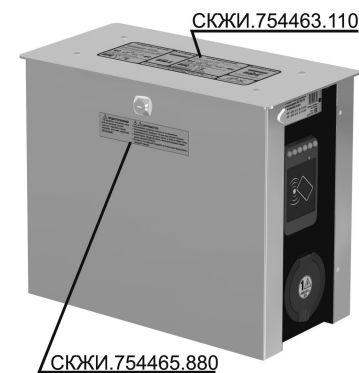
Рисунок 7 – Места расположения этикеток
