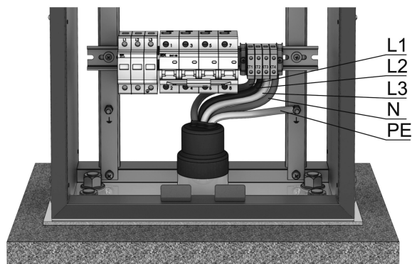
Рисунок 6 – Подключение станции к сети энергоснабжения
