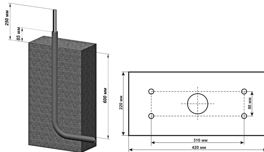
Рисунок 4 – Конфигурация фундамента для монтажа
