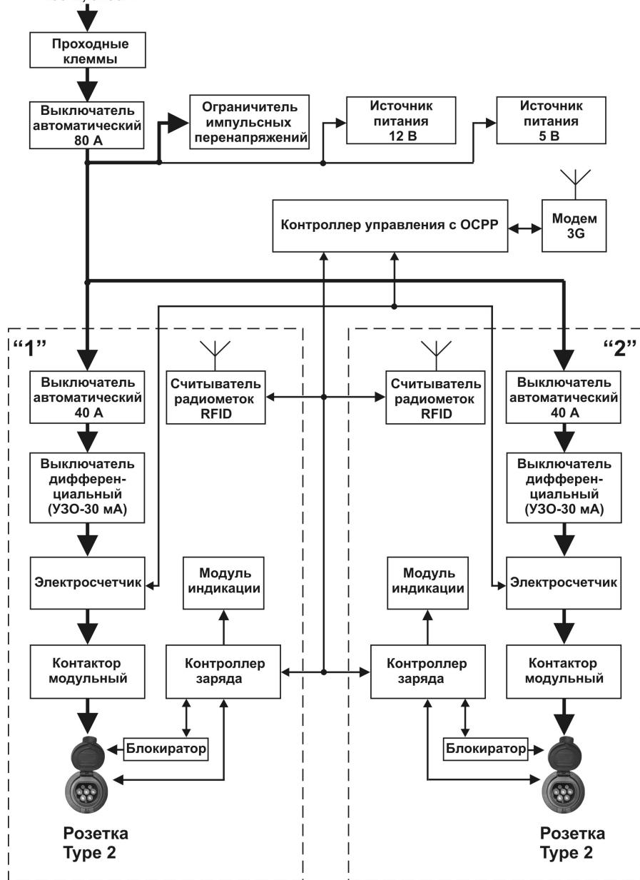
Рисунок 3 – Структурная схема станции ЕС-301-48
