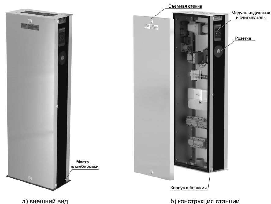
Рисунок 2 – Внешний вид и конструкция станции
