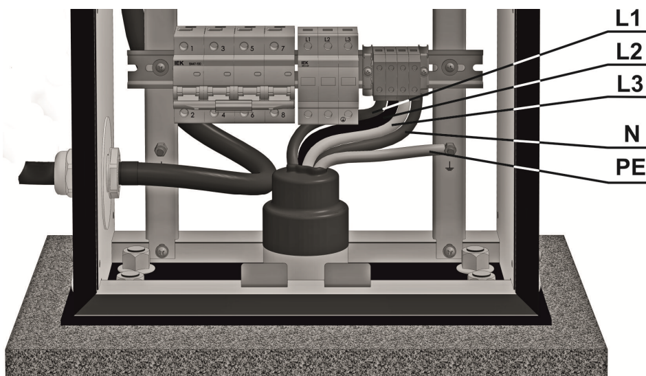
Рисунок 6 – Подключение станции к сети энергоснабжения
