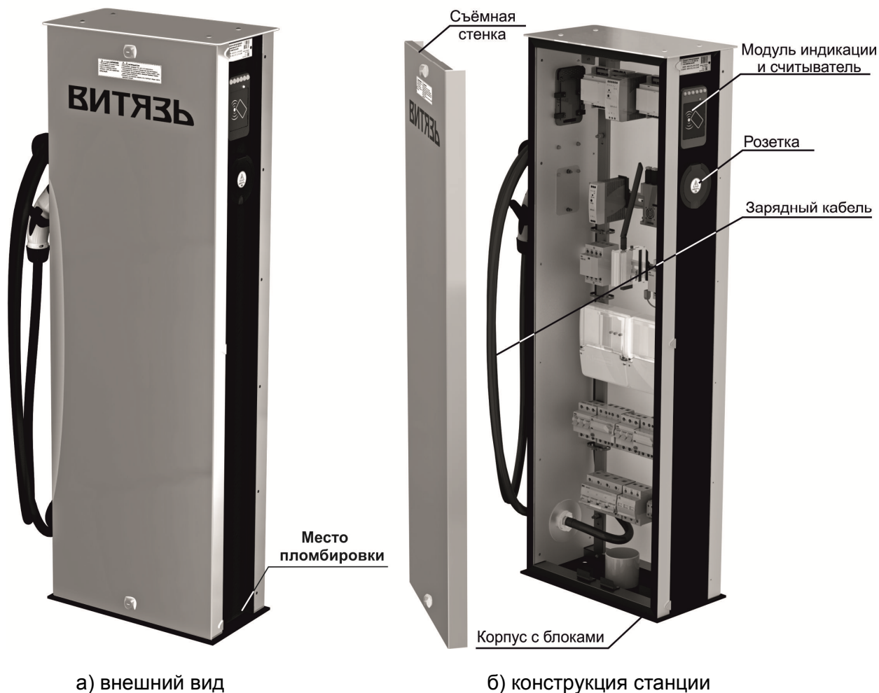
Рисунок 2 – Внешний вид и конструкция станции
