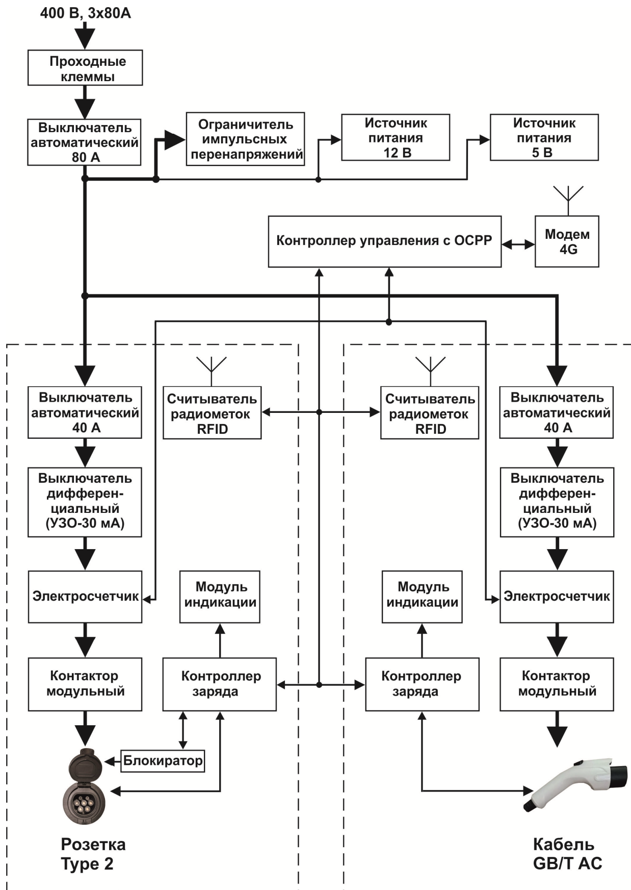
Рисунок 3 – Структурная схема станции EC-301-58
